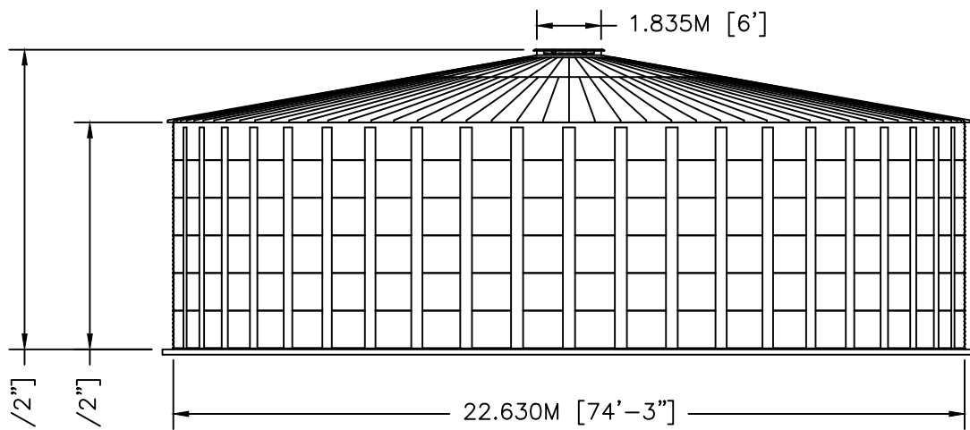
ELEVATION
