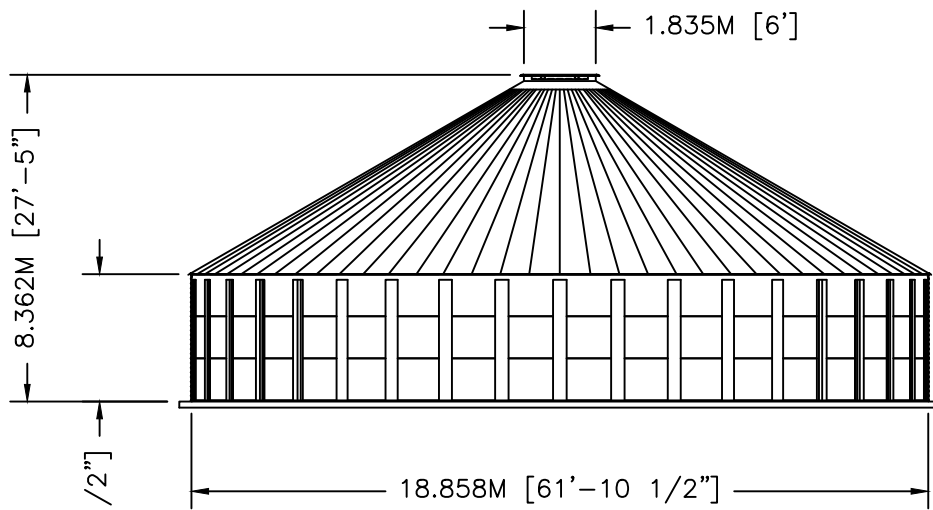
ELEVATION
