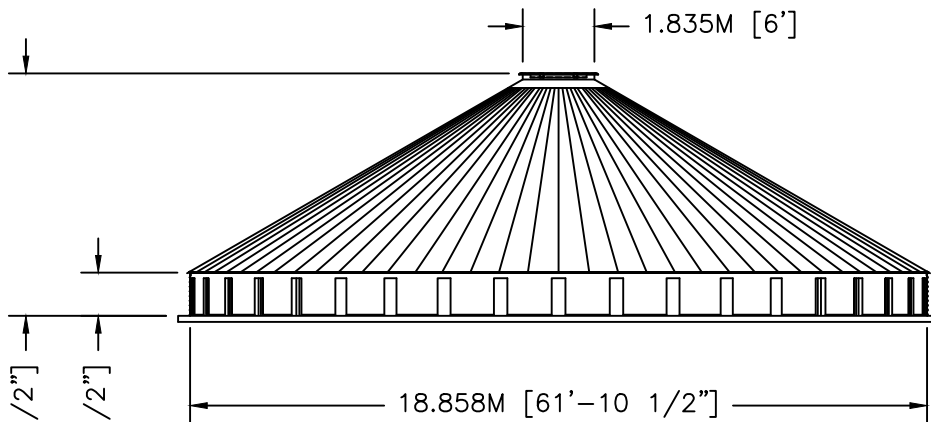
ELEVATION
