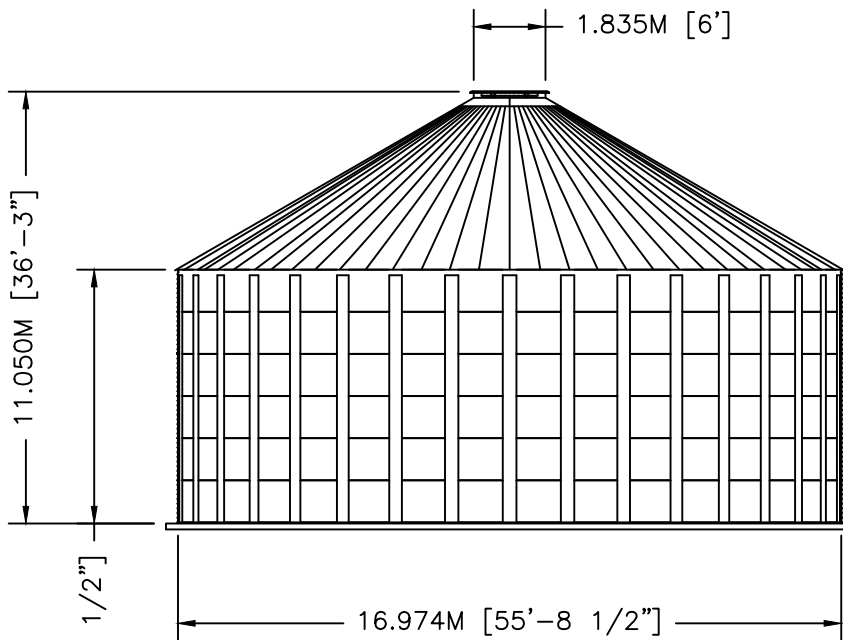
ELEVATION
