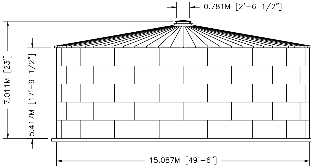
ELEVATION
