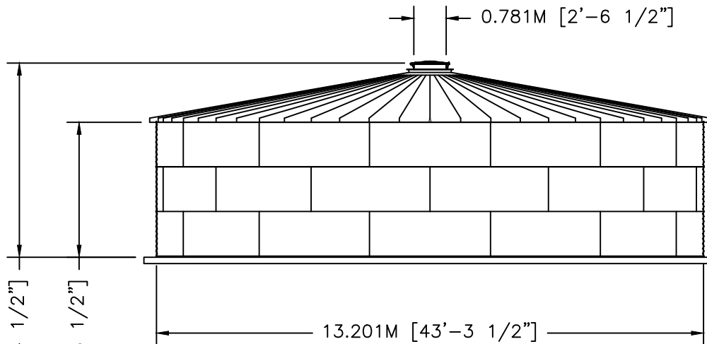
ELEVATION
