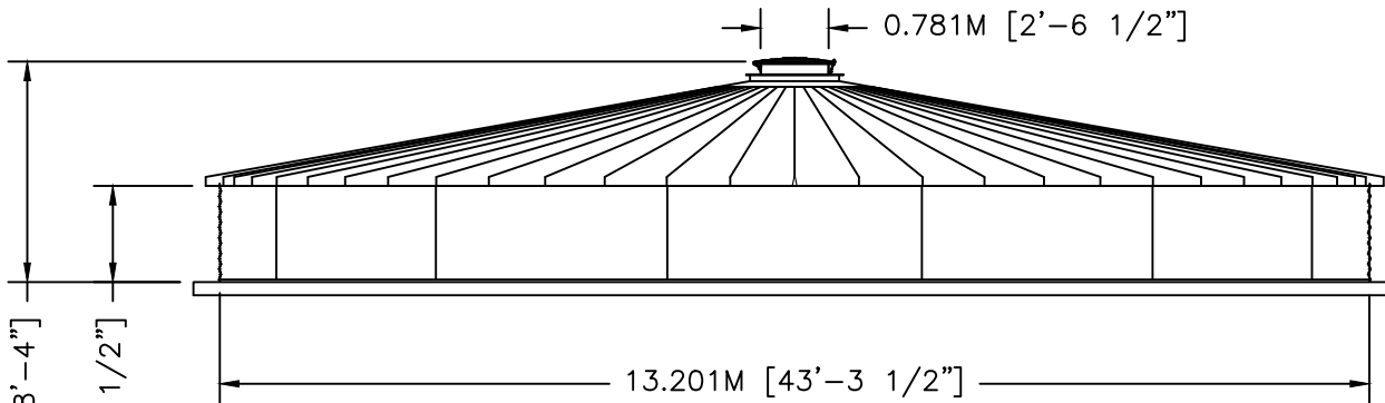
ELEVATION
