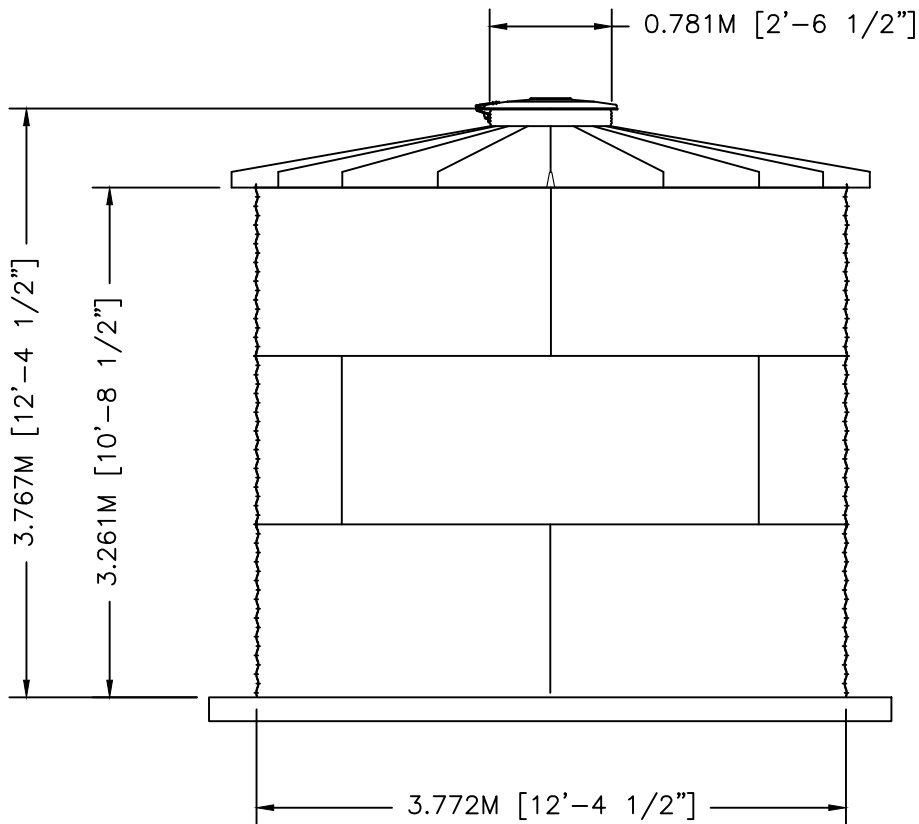
ELEVATION
